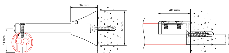
Wandmontage met inkortbare afstandsteun 4217-101, steun kan ingekort worden tot 50 mm
