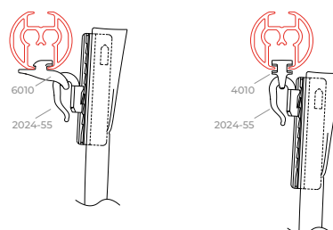
Hoofdje met voorsprongglijder 6010 breedte 15 mm
