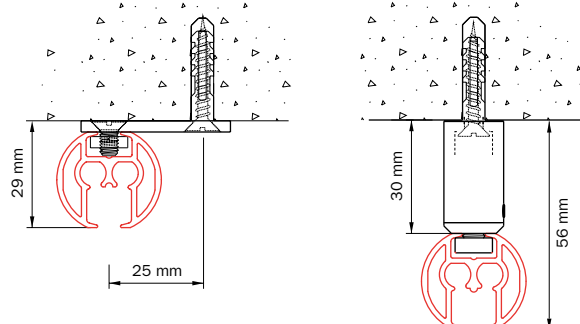
Plafondmontage 5100 met plafondsteun 5135
