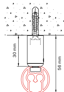
Plafondmontage 5100 met plafondklos 4254
