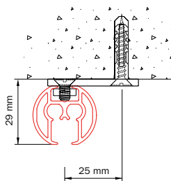
Plafondmontage 5100 met plafondsteun 5135
