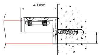
Wandmontage 5100 met dagsteun 5149
