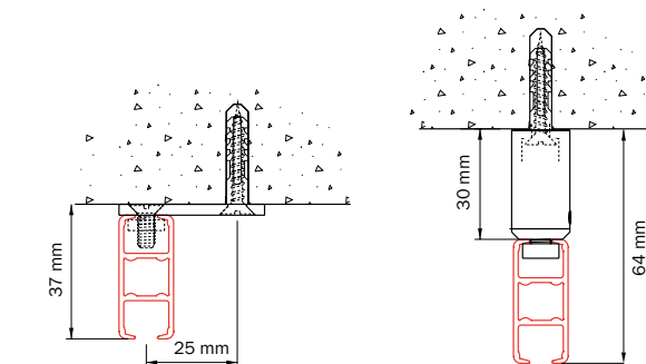
plafondmontage 4100 met plafondsteun 4135
