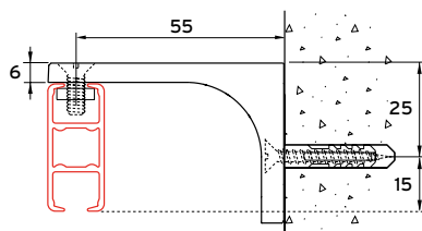
wandmontage met muurbeugel 4140
