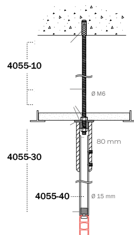
Plafondmontage 4100 aan pendel 4055-40 met montageset 4055-30, pendel aan draadeindset 4055-10.
