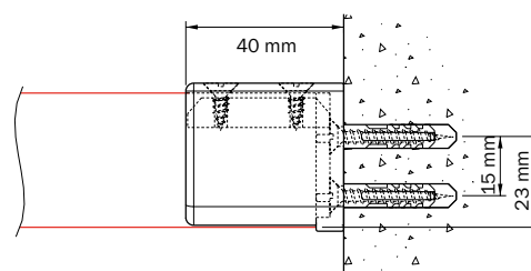
wandmontage 4100 met dagsteun 4149
