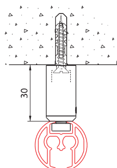
plafondmontage 5100 met plafondklos 4254
