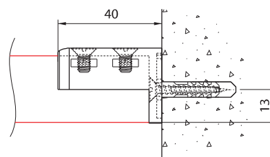
wandmontage 5100 met dagsteun 5150
