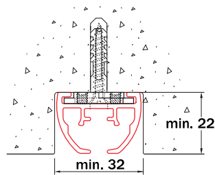
blindmontage b.v. in groef met steun 6055-2000 bij bochten: freesgroef maken op basis van geleverde rail
