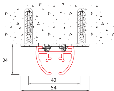
plafondmontage met plafondsteun 6055-100
