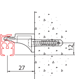
wandmontage met wandsteun 5351
