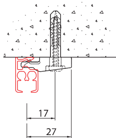
wandmontage met plafondsteun 5350
