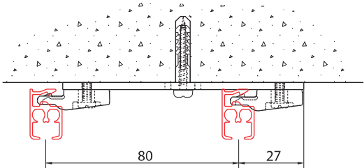
plafondmontage met dubbeldrager 2216-53 en plafondsteun 5350
