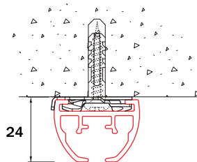
plafondmontage met spanner 6050
