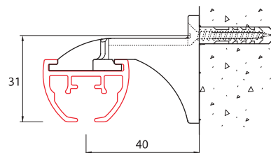
wandmontage met wandsteun 6051
