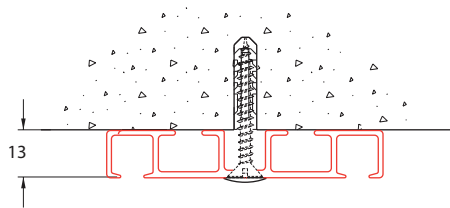
plafondmontage 4540 met 4514-WD schroef met wit afdekdopje
