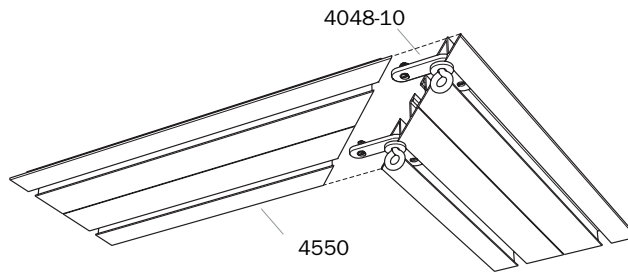
Voorbeeld van een haakse verbinding bij een meerspoorprofiel.
