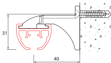
wandmontage met wandsteun 6051
