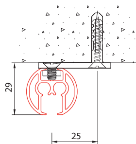
plafondmontage 5100 met plafondsteun 5135
