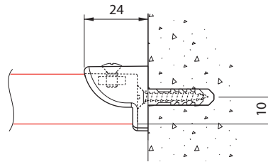
wandmontage 4200 met dagsteun 4249
