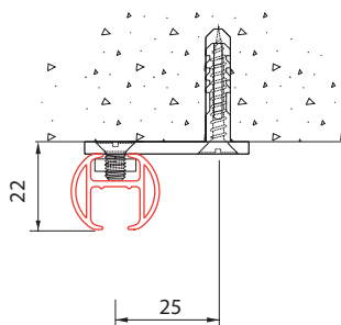
plafondmontage 4200 met plafondsteun 5153
