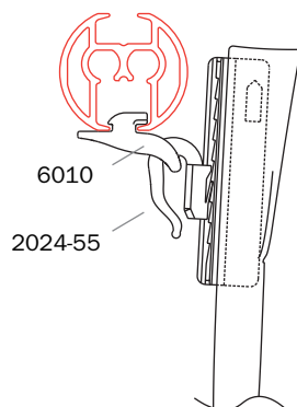
hoofdje met voorspronglijder 6010
