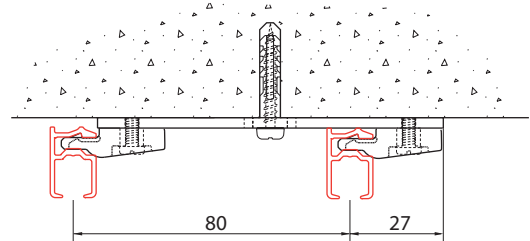
plafondsteun met dubbeldrager 2216-53 en plafondsteun 5350
