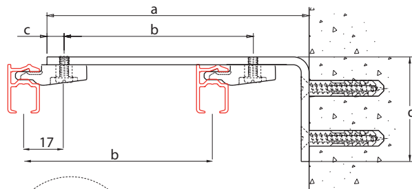
detail voorzijde afstandsteun
