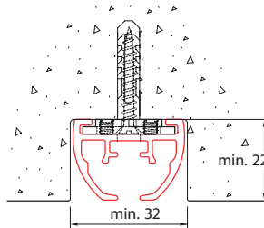
blindmontage b.v. in groef met steun 6055-2000 bij bochten: freesgroef maken op basis van geleverde rail
