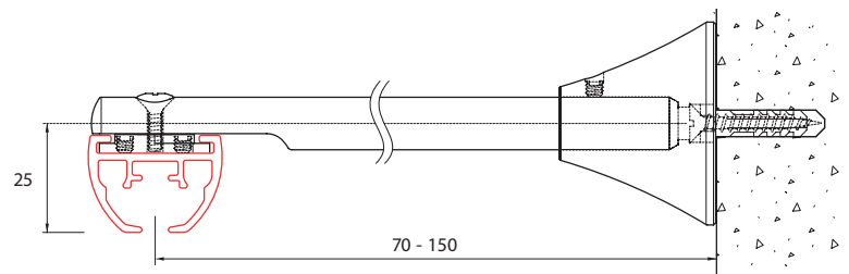
wandmontage met inkortbare afstandsteun 6057
