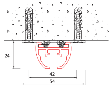
plafondmontage met plafondsteun 6055-100
