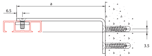
wandmontage 4520 met afstansteun 4515-10
