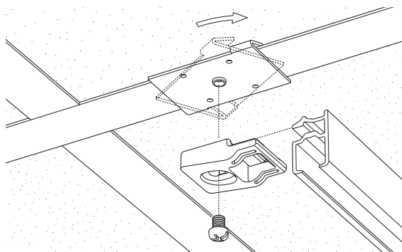
montage aan systeemplafond d.m.v. klemsteun
