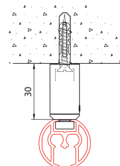
plafondmontage 5100 met plafonklos 4254
