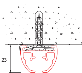
plafondmontage met spanner 6050
