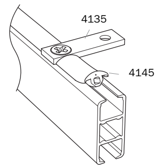
plafondmontage met plafondsteun 4135 en stofstrip 4145 ter afdichting van de kier
