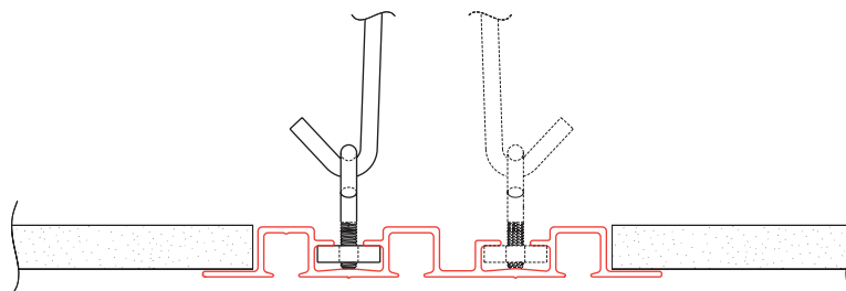
montage 4560 in systeemplafond met 4555-SH
