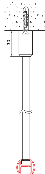
plafondmontage met 4255
