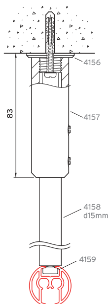
plafondmontage met 4155
