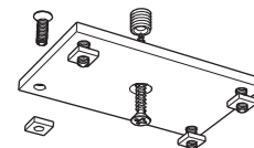
4116 (t.b.v. 4100) 5116 (t.b.v. 4200 & 5100) dubbeldrager
