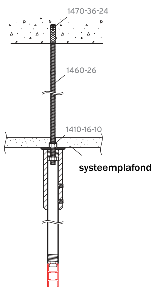
plafondmontage met 4155 bij systeem- plafond met bronzen plug en draaideind
