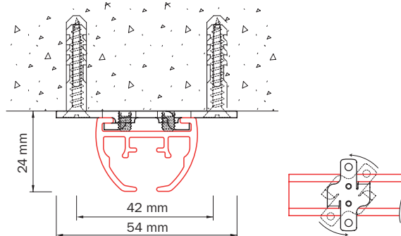
Plafondmontage met plafondsteun 6055-1000
