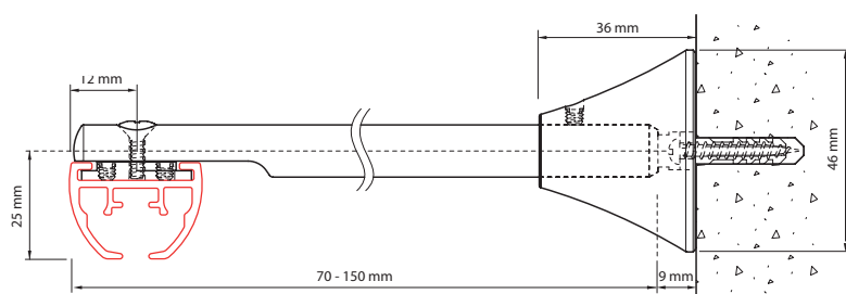
Wandmontage met inkortbare afstandsteun 6017
