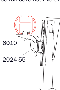
Hoofdje met voorsprongglijder 6010 breedte 15 mm
