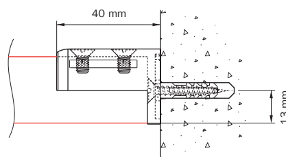
Wandmontage 5100 met dagsteun 5149
