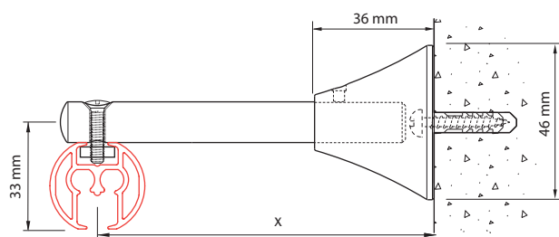
Wandmontage met inkortbare afstandsteun 4217-101, steun kan ingekort worden tot x = 50 mm
