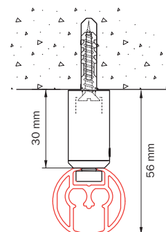
Plafondmontage 5100 met plafondklos 4254
