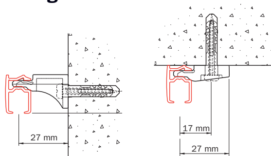
Wandmontage met wandsteun 5351
