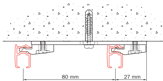
Plafondsteun met dubbeldrager 2216 en plafondsteun 5350
