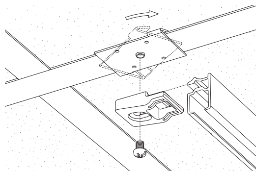
Montage aan systeemplafond d.m.v. klemsteun, deze toepassing is niet geschikt voor zware gordijnen.
