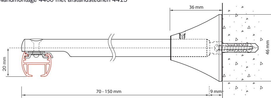
Wandmontage 4400 met afstandsteunen 4415
