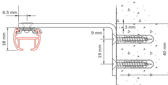
Wandmontage 4400 met afstandsteunen 4415
