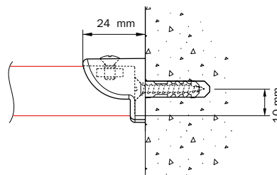
Wandmontage 4200 met dagsteun 4249
