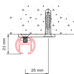
Plafondmontage 4200 met plafondsteun 5135
