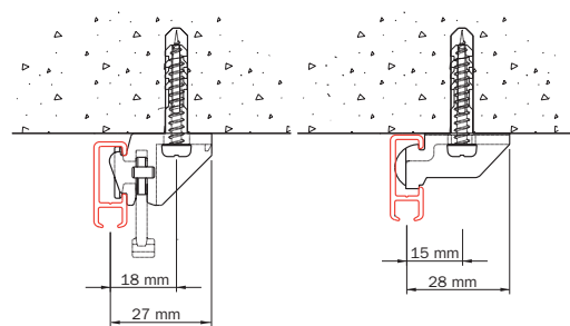
Plafondmontage met 7450.
