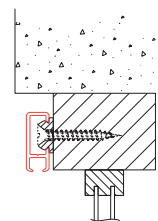
Montage op kozijn met 2254.
