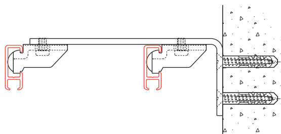
Wandmontage met 2015 wandsteunen.
