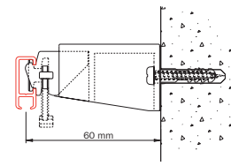
Wandmontage met 7451.
