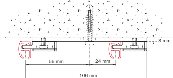
Voor goede parallelle plaatsing: montage met dubbeldrager 2216 en plafondsteunen 2150.
