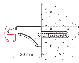
Wandmontage met wandsteun 2151.
