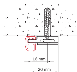
Plafondmontage met plafondsteun 2150.
