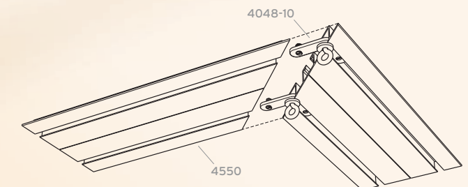
Voorbeeld van een haakse verbinding bij een meerspoorprofiel.
