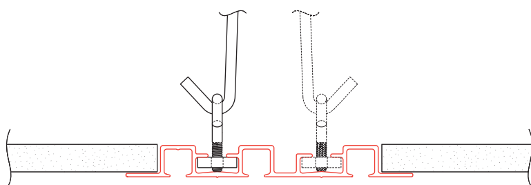
montage 4560 in systeemplafond met 4555-SH
