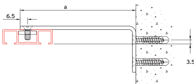
wandmontage 4520 met afstandsteun 4515-10
