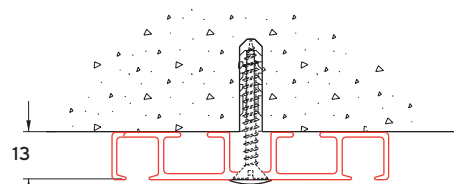
plafondmontage 4540 met 4514-WD schroef met wit afdekopje
